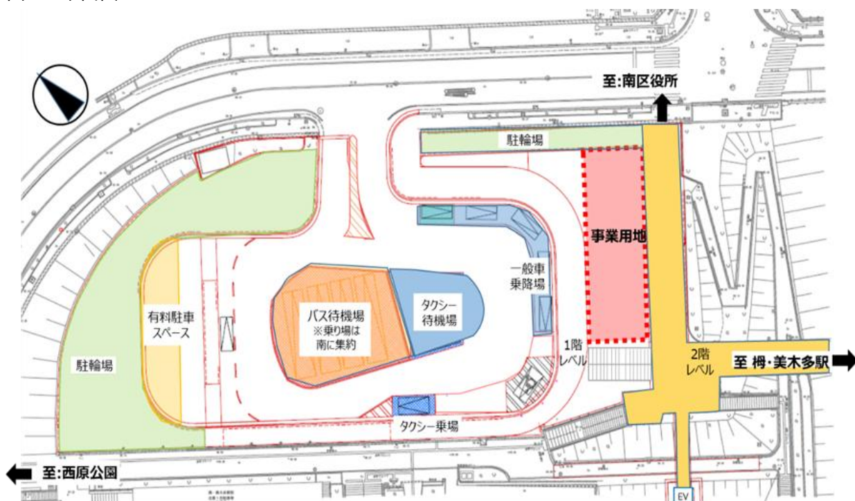
図 2 平面図
