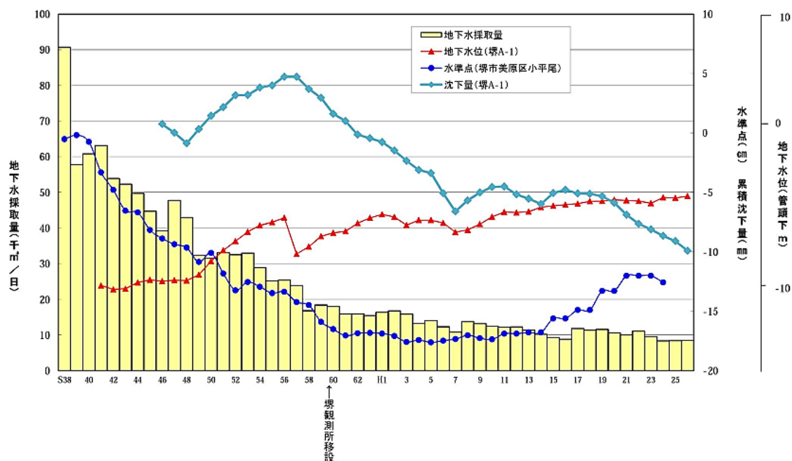
図 3. 1-8 堺市における地下水採取量と地下水位・累積沈下量の相関
