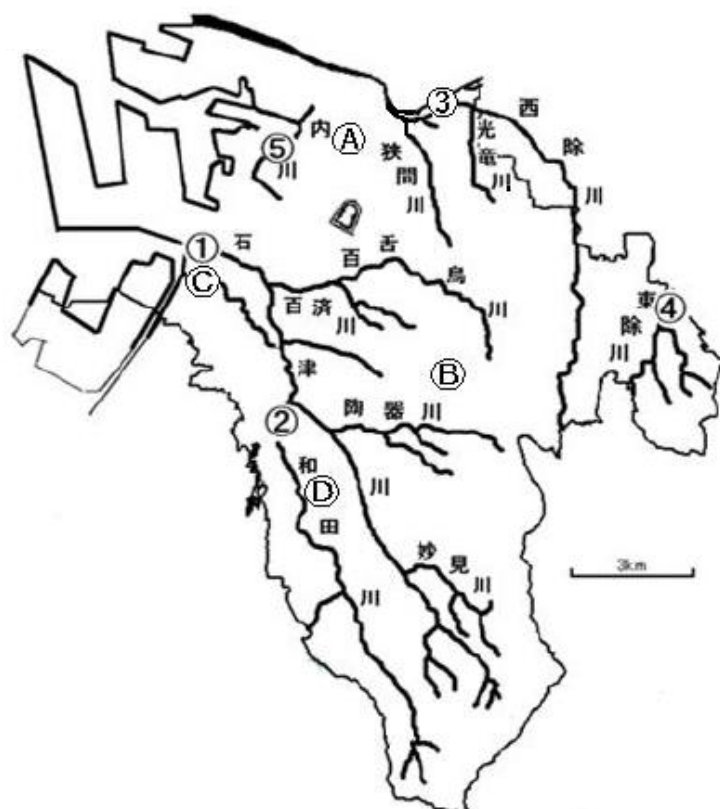
図 3.2-6 水質及び底質中のダイオキシン類調査地点
