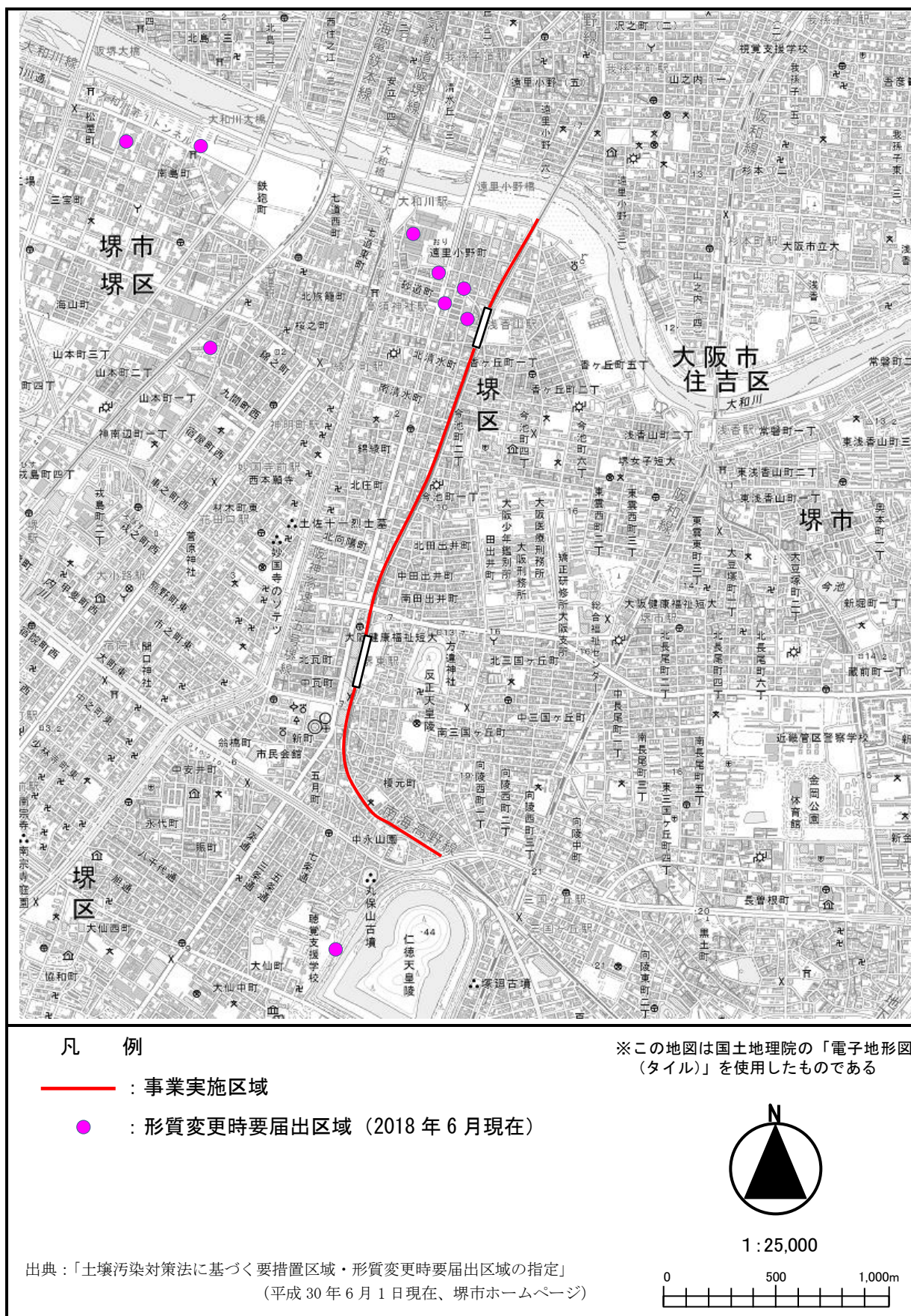
図 3.2-7 事業実施区域周辺の土壌汚染地区
