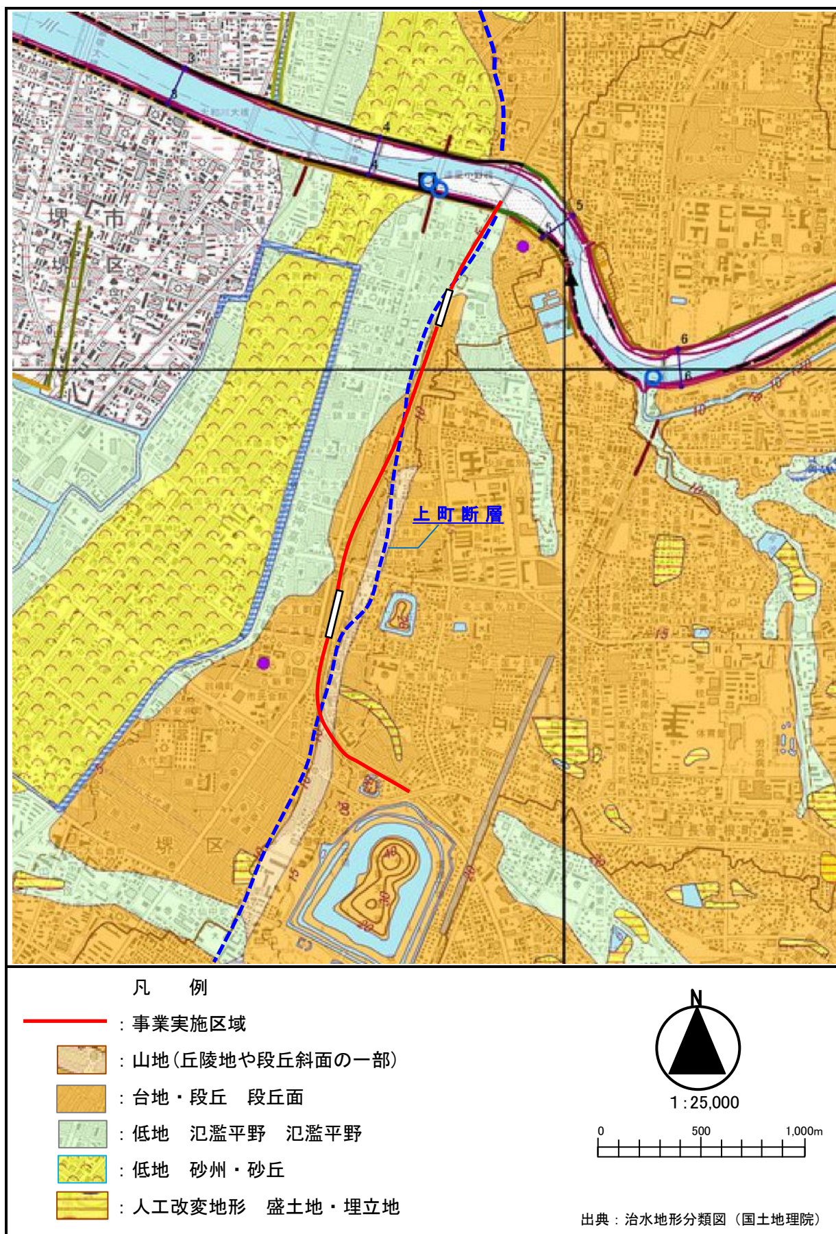
図 3.3-3 事業実施区域周辺の治水地形分類図
