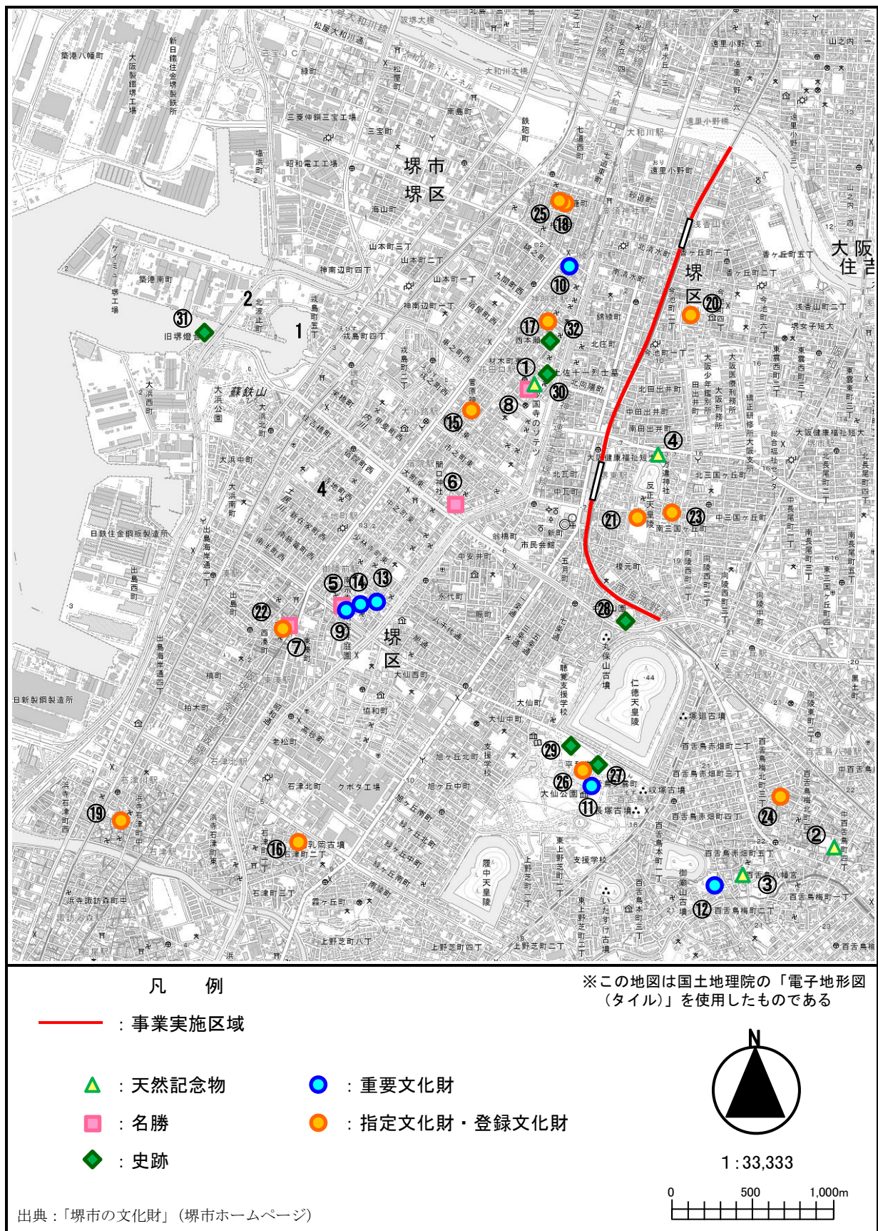
図 3.4-2 事業実施区域周辺の指定文化財の分布状況
