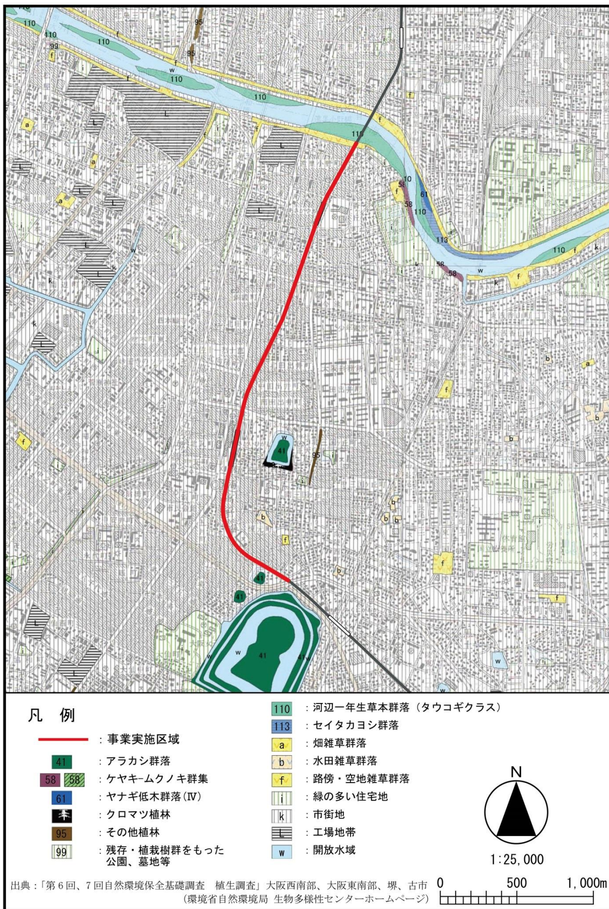
図 3.3-6 事業実施区域周辺の植生図
