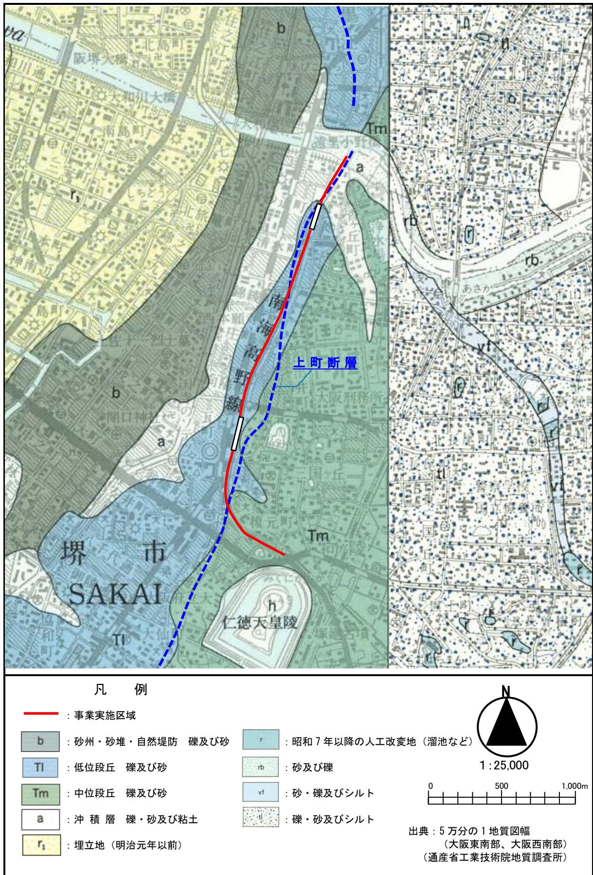
図 3. 3-4 事業実施区域周辺の表層地質図
