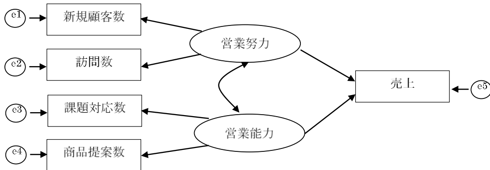
＜パス図の例＞
