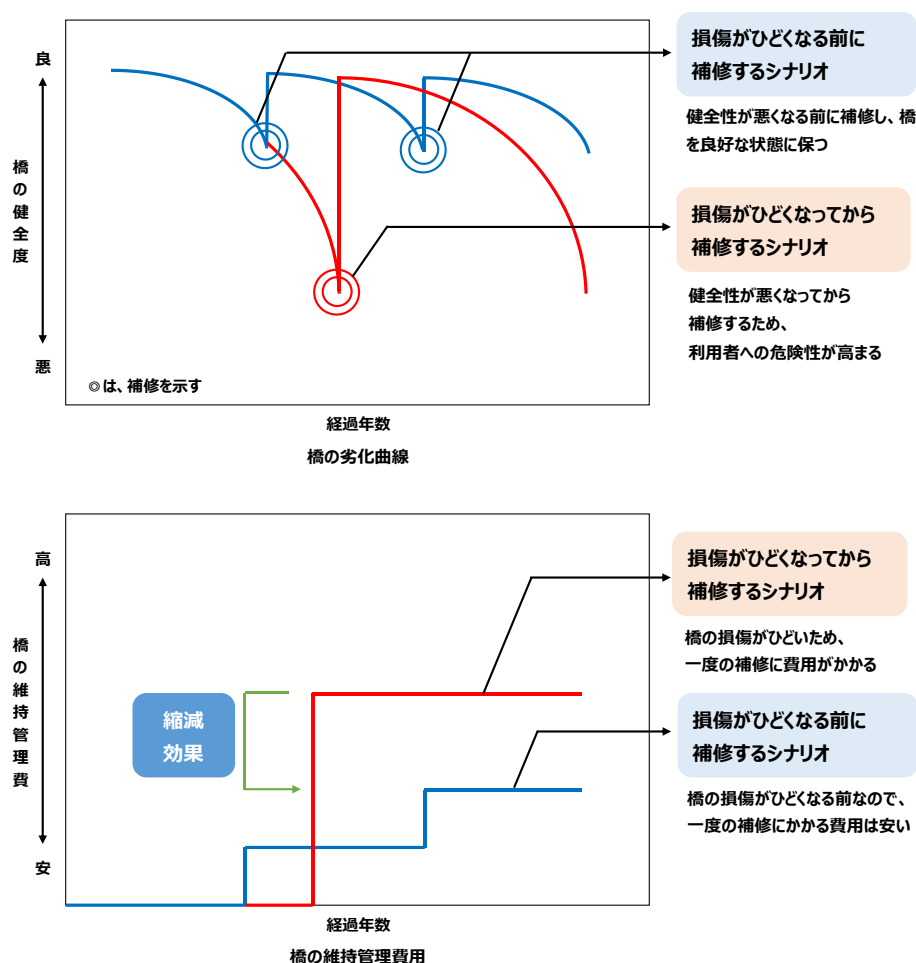
図表 4-2-3 橋りょうを例としたライフサイクルコスト削減の考え方
