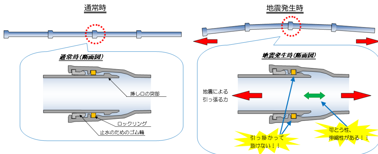
図表 4-6-3 耐震管のイメージ
