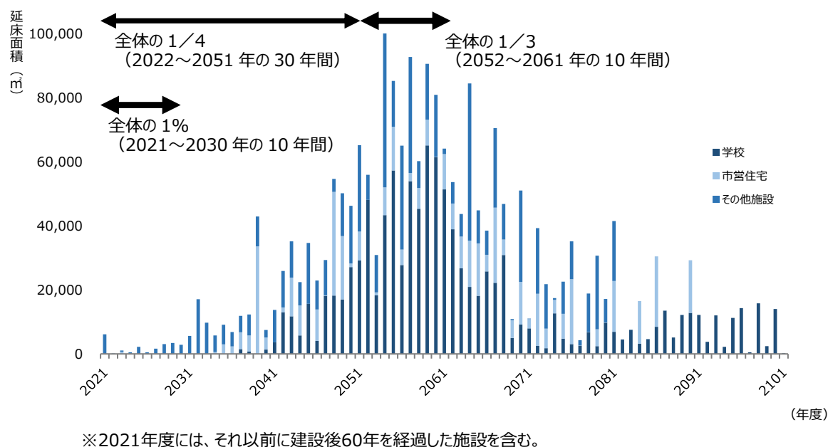
図表 3-2-7 長寿命化後の耐用年数を迎える施設の延床面積
