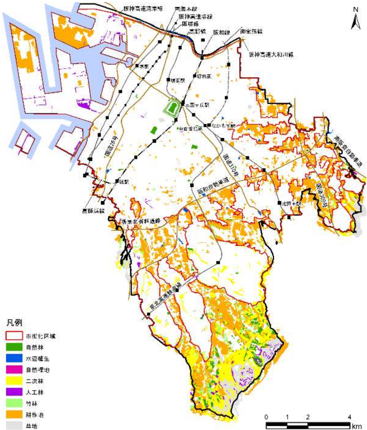
植生の状況
