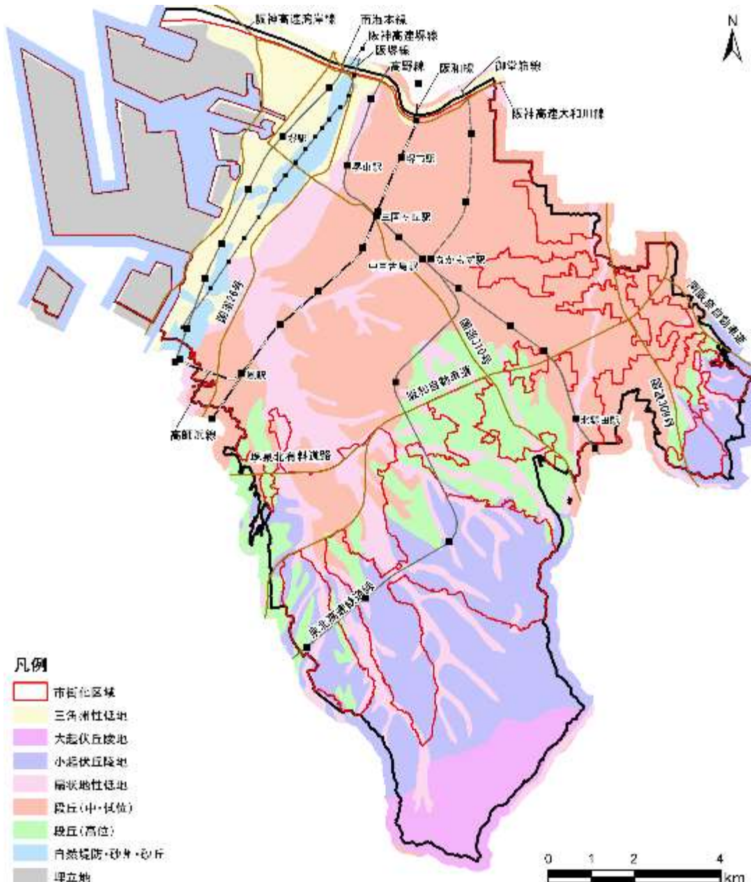
地形区分図
