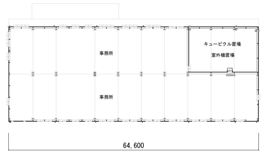
3階平面図
