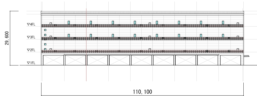
東立面图
