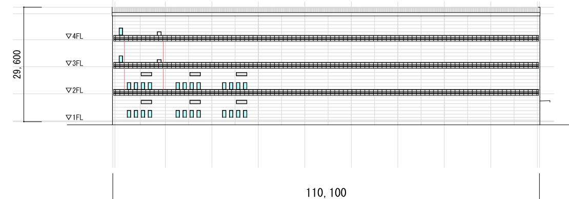
西立面图
