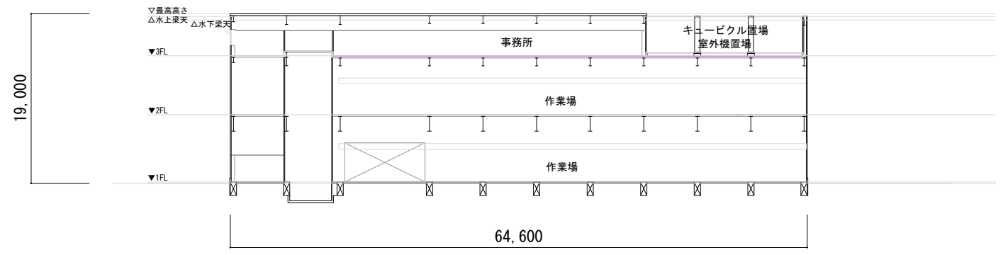
断面図
