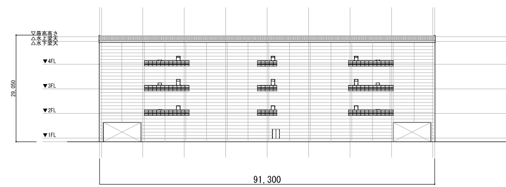
西立面图
