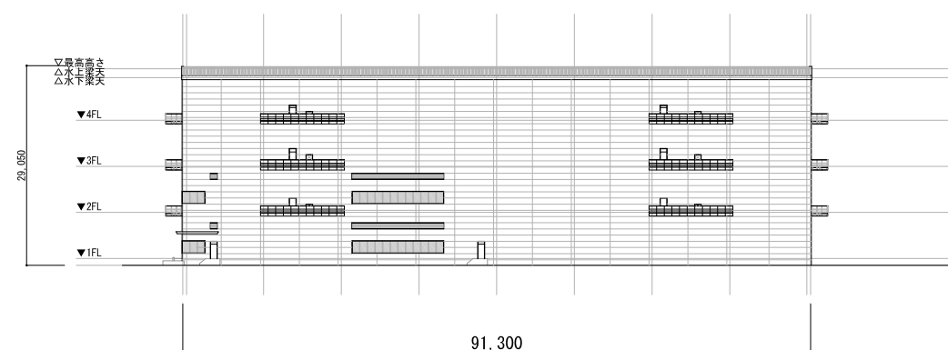
東立面图
