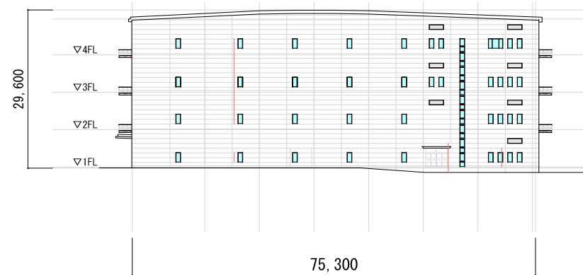
北立面图
