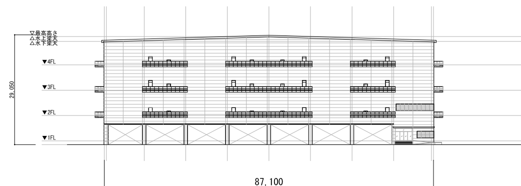
南立面图
