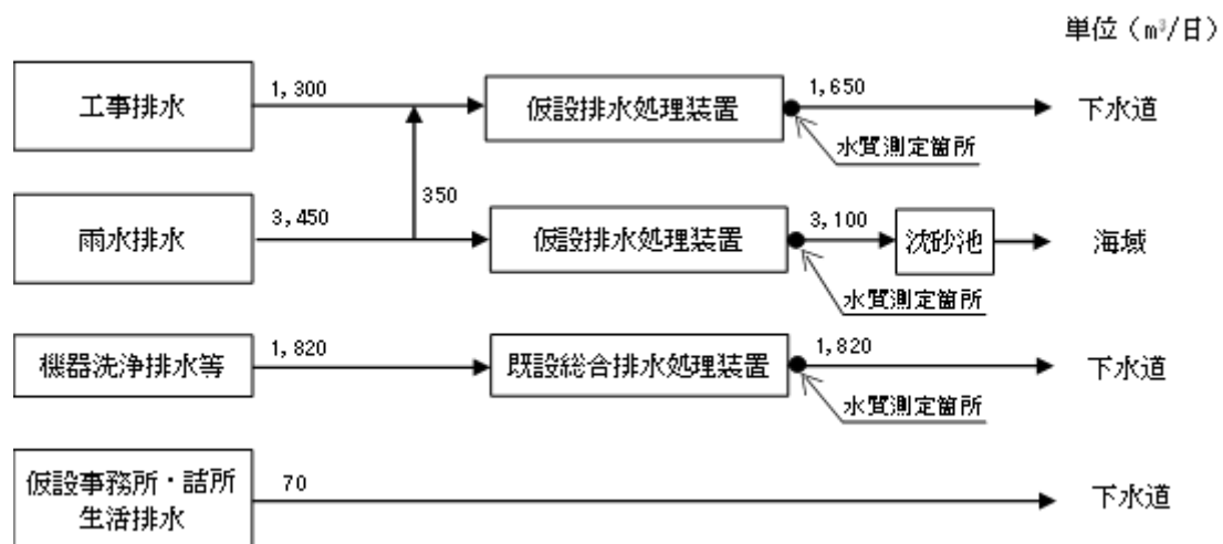
図Ⅱ-3-13 工事中の排水に係る処理フロー
