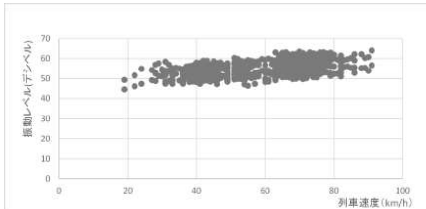
図 A4 地点における速度と振動レベル散布図
