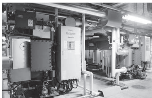
吸収式冷温水発生機
