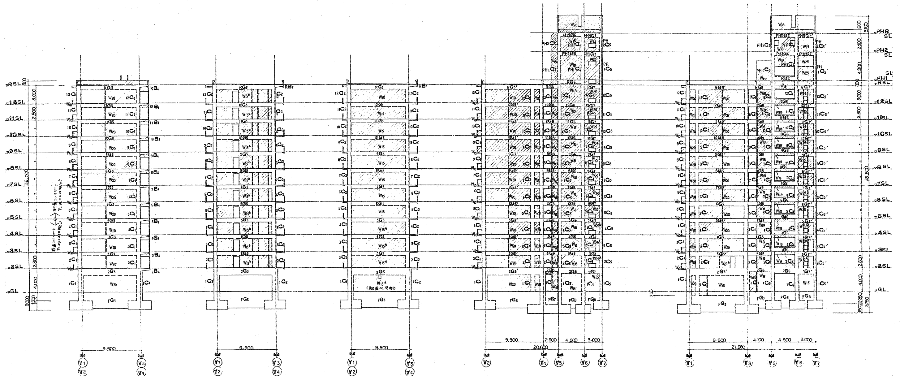
X1・X14通軸組図 S=1/400
