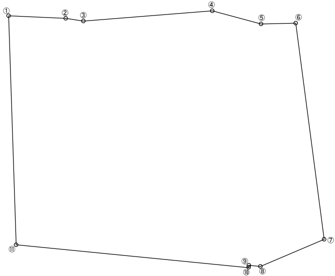
敷地面積求積図 1:800
