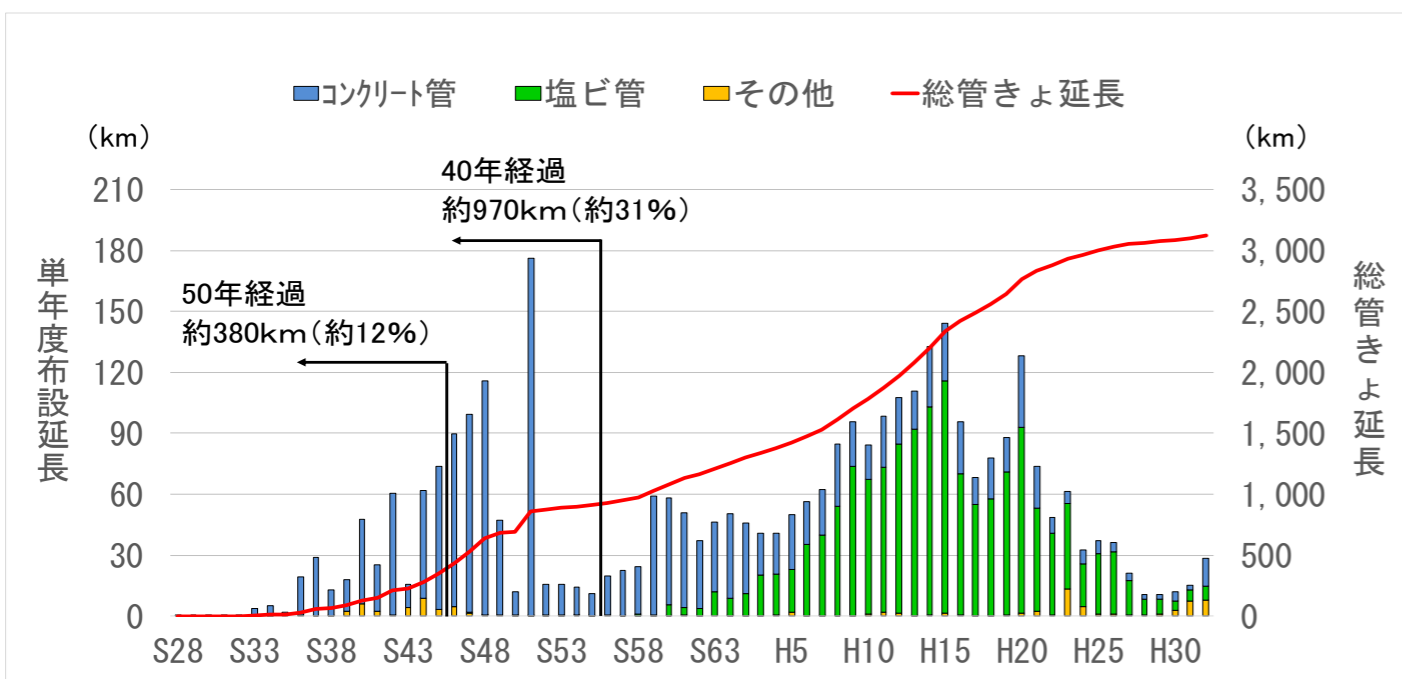
管種別の管渠延長
