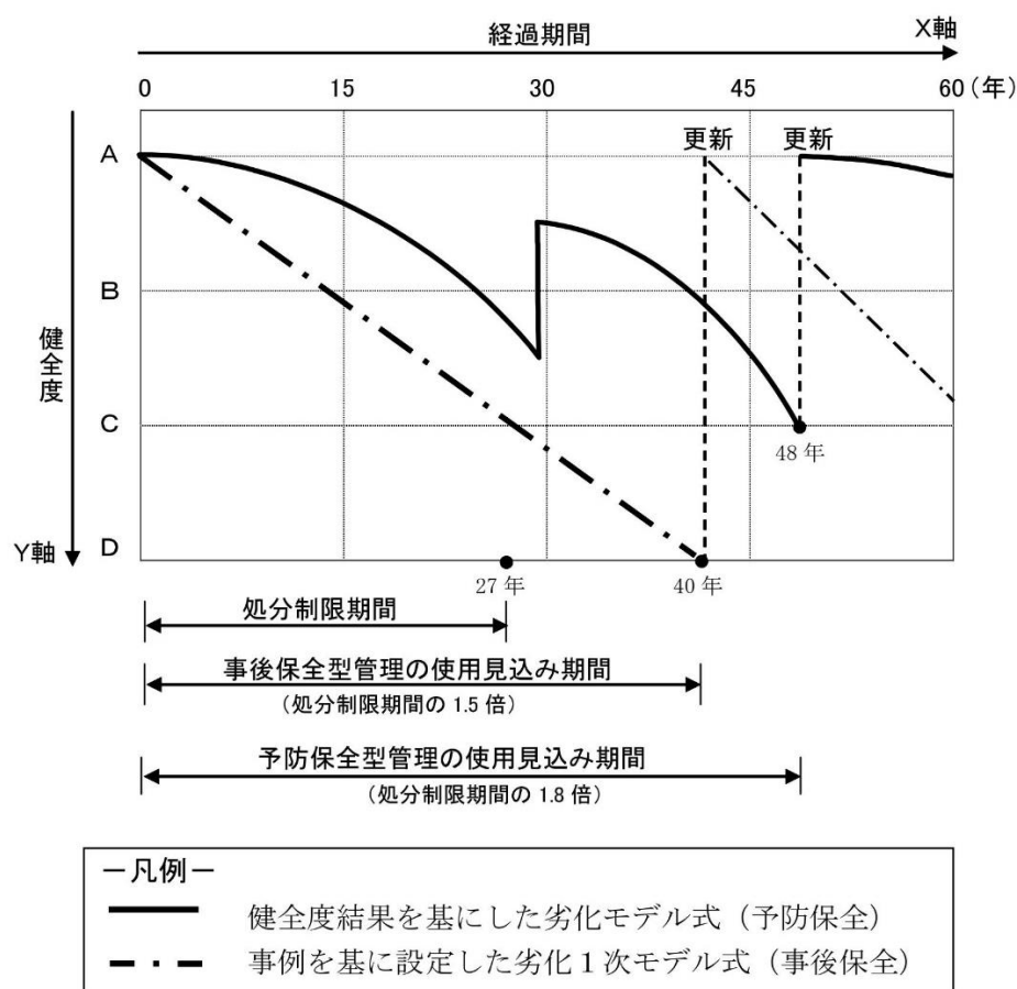
図 更新見込み年度の概念図（処分制限期間が 20 年以上～40 年未満の施設）
