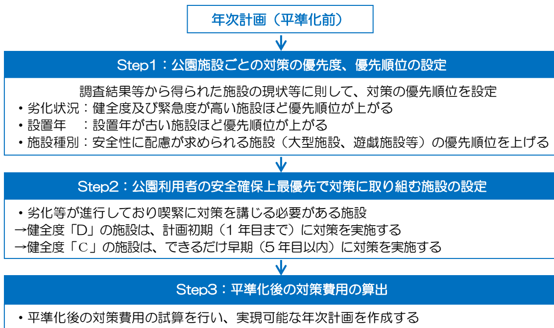
図 平準化方針
