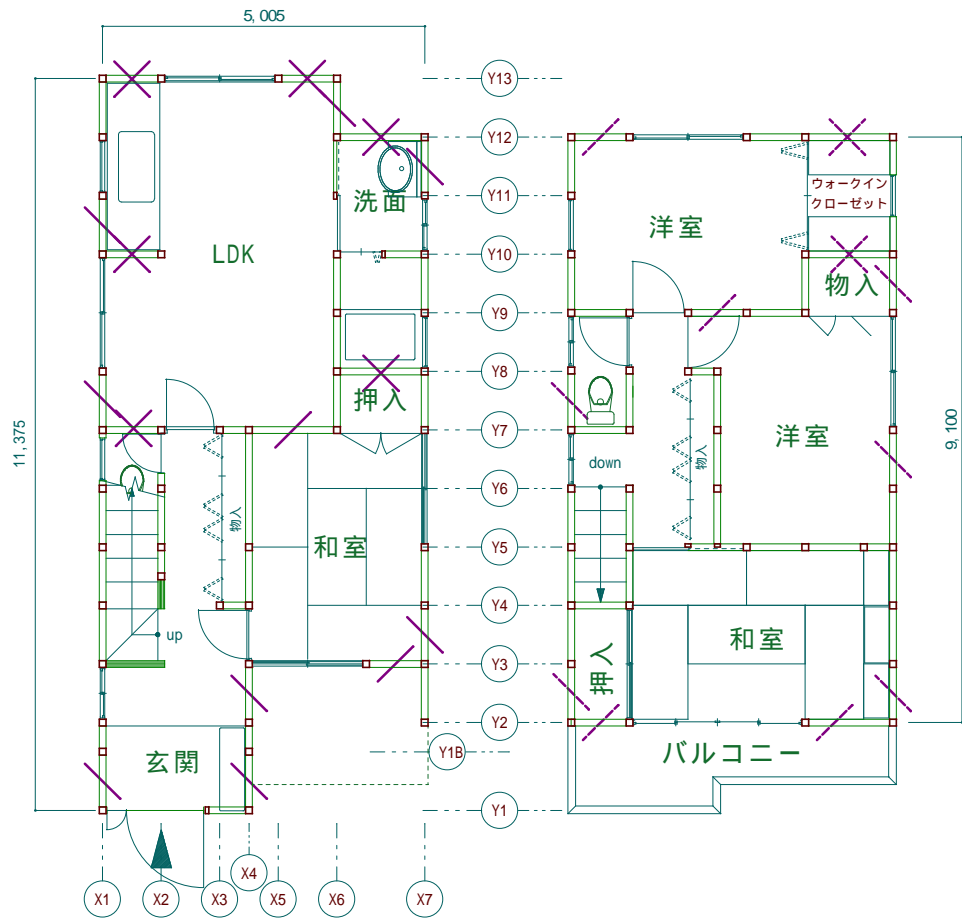
1F平面図
