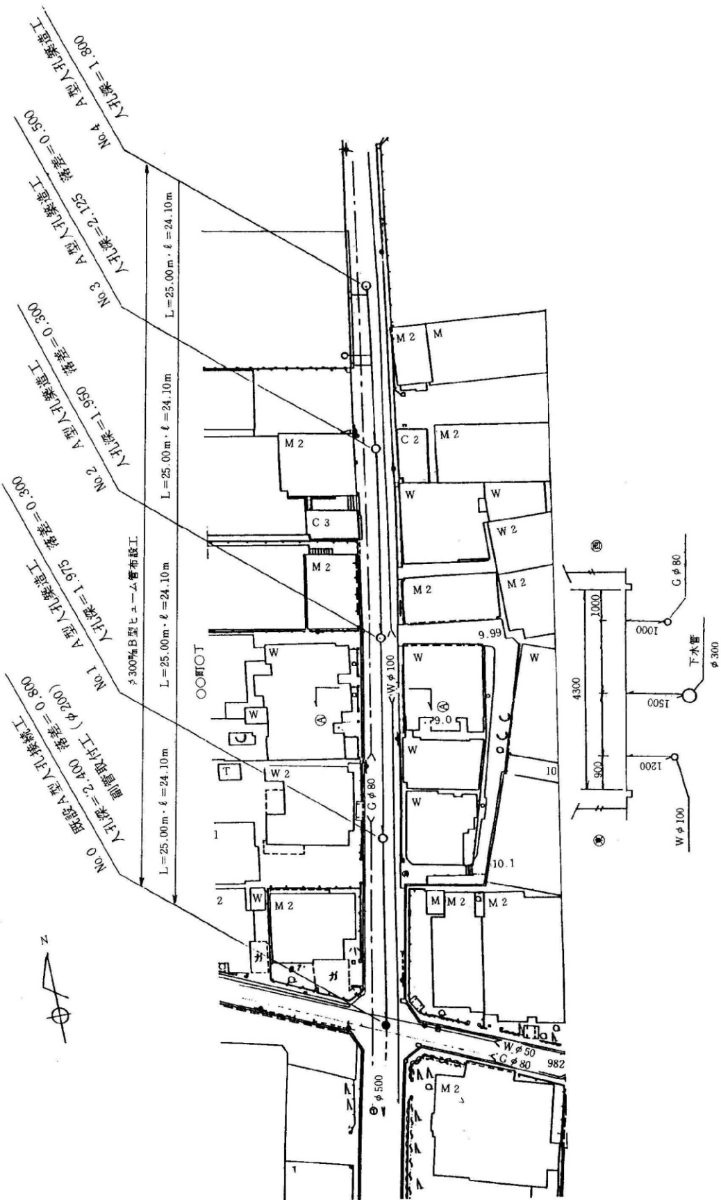
下水道計画平面図
