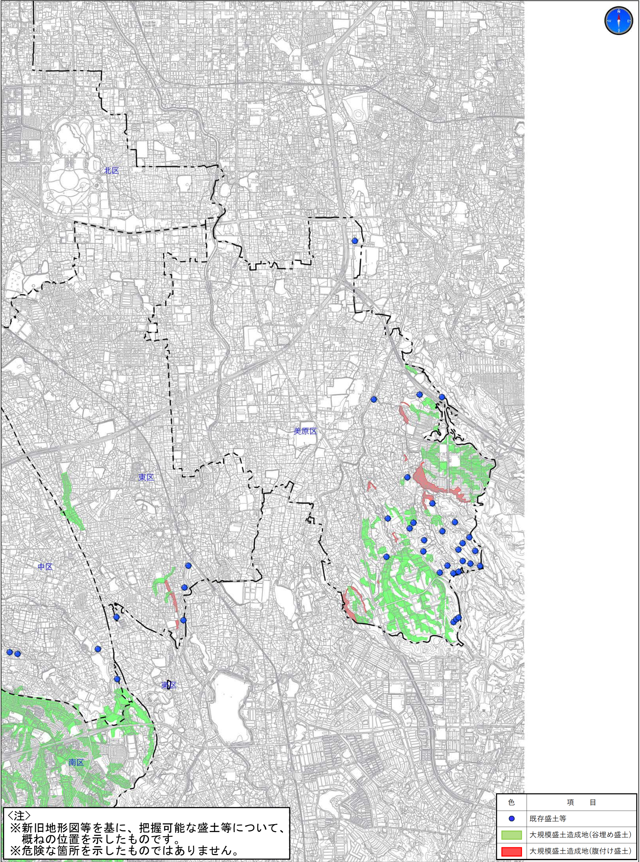
既存盛土等位置図（美原区）
