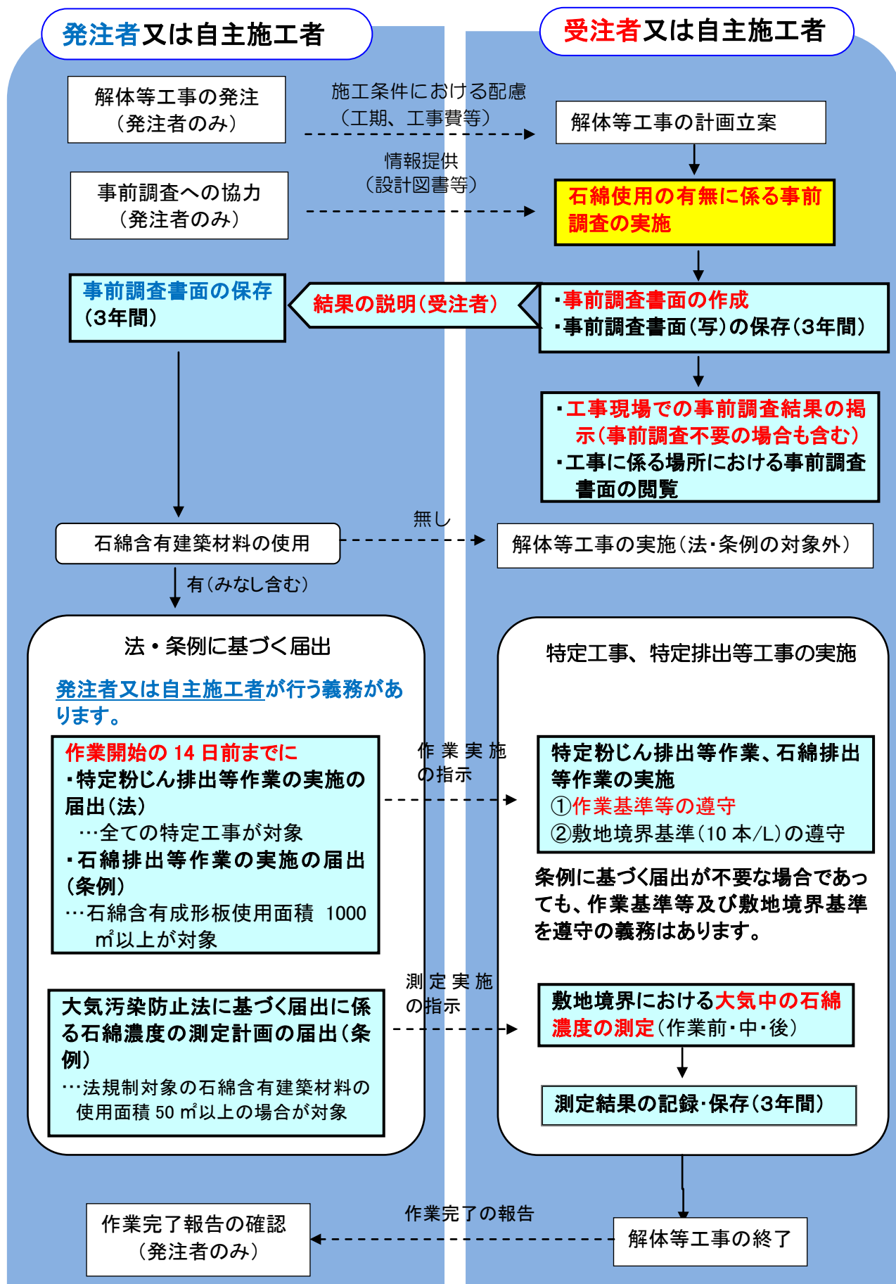
図1 法及び条例に基づく石綿(アスベスト)飛散防止対策のフロー
