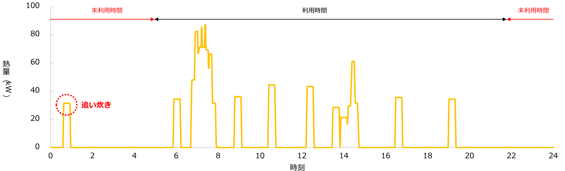
温水ボイラの平均熱出力
