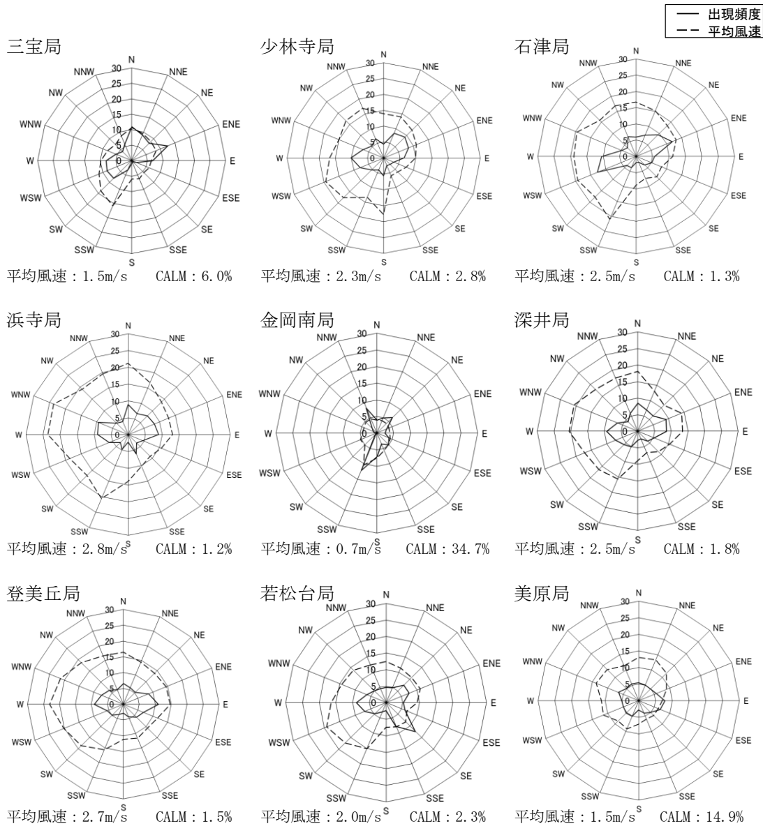
図9-1 平成30年度 年間風配図 (一般環境大気測定局)
