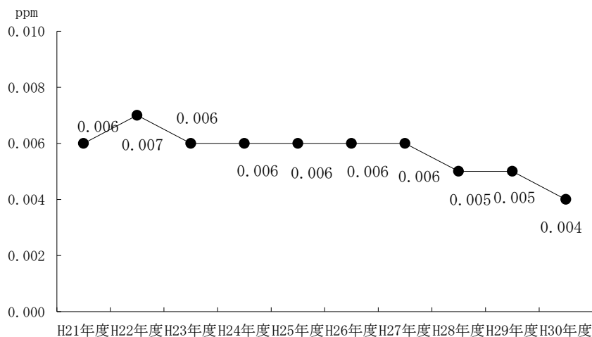
図5-1 二酸化硫黄 年平均値の推移 (市内平均値)
