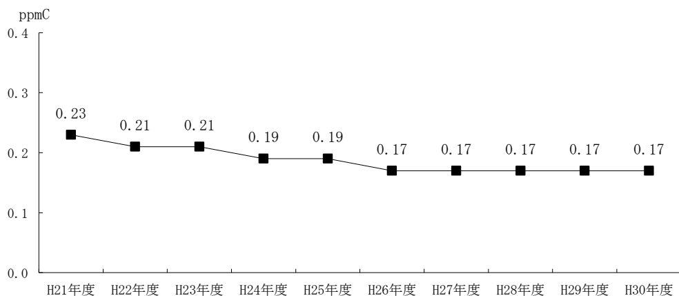
図7-1 非メタン炭化水素 年平均値の推移
