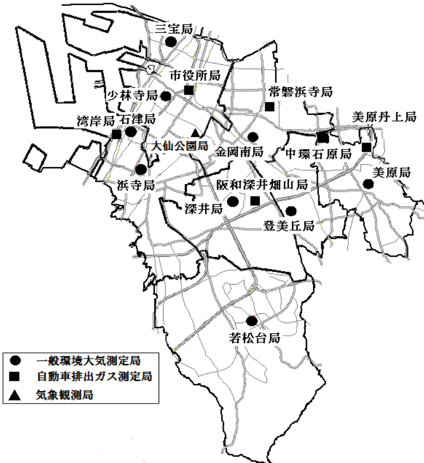
図 1 - 1 平成30年度 測定局地点図
