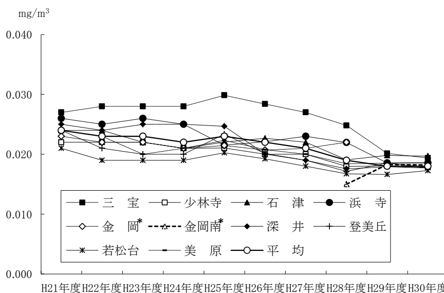
図3-2 浮遊粒子状物質 年平均値の推移（一般環境大気測定局）
