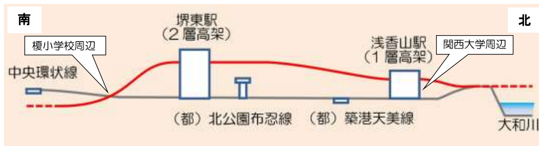
図 I -4-7 縦断概略図
