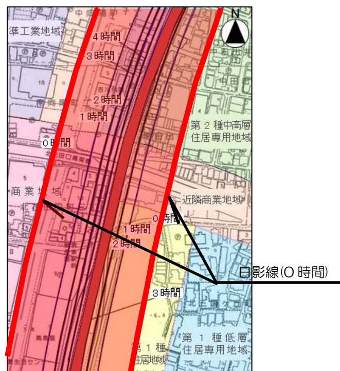
北花田口跨線橋付近における高架構造物（17m）の等時間日影線図 (冬至日における8時～16時における日影の発生時間を示す。)
