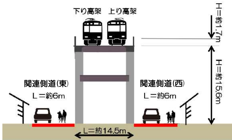
図 I-4-4 標準断面図（2層高架構造）
