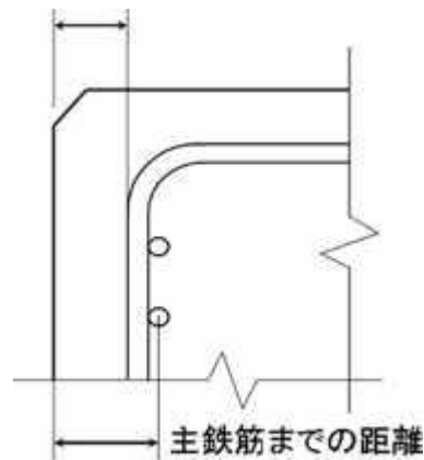
図1-3-1 鉄筋のかぶり
