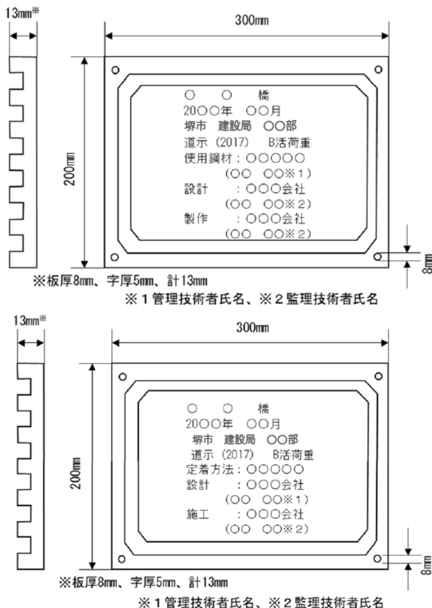
図 3-2-2 銘板の寸法及び記載事項
