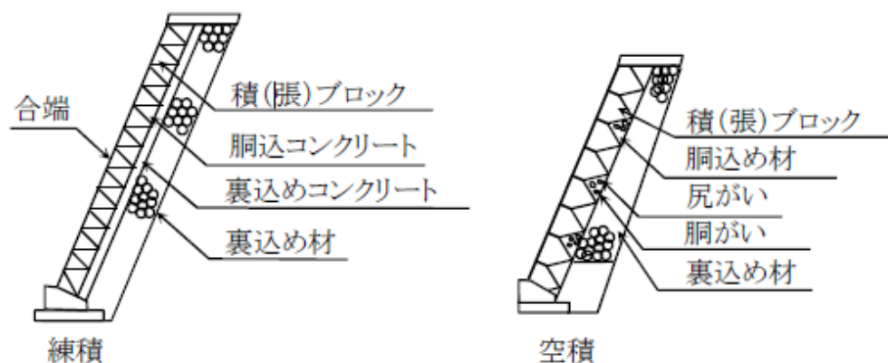
図 3-2-5 コンクリートブロック工
