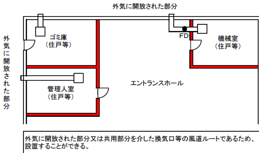
第3-21図 (認められる設置例)
