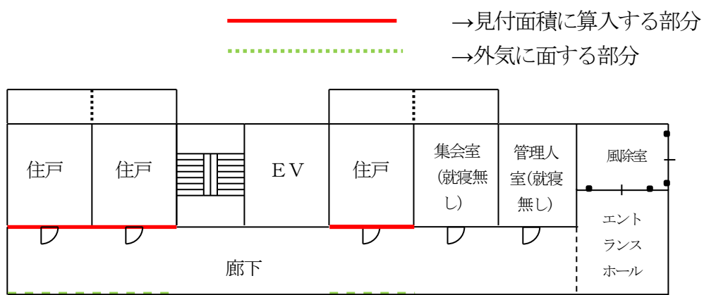
第4-18図 (避難階における開放性検証の対象)
