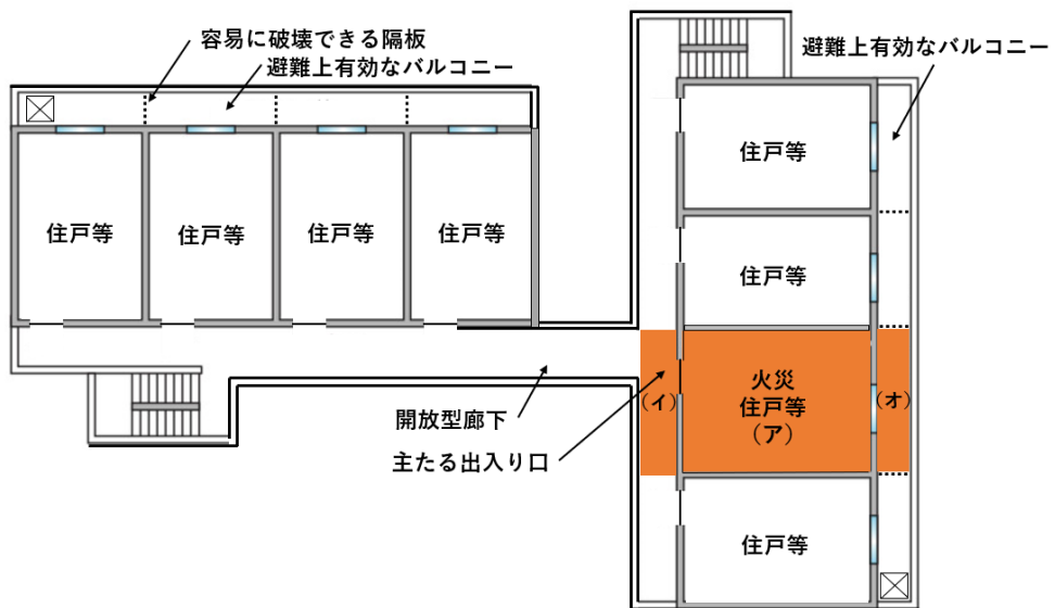
第4-4図 (廊下型特定共同住宅等 (T字型))
