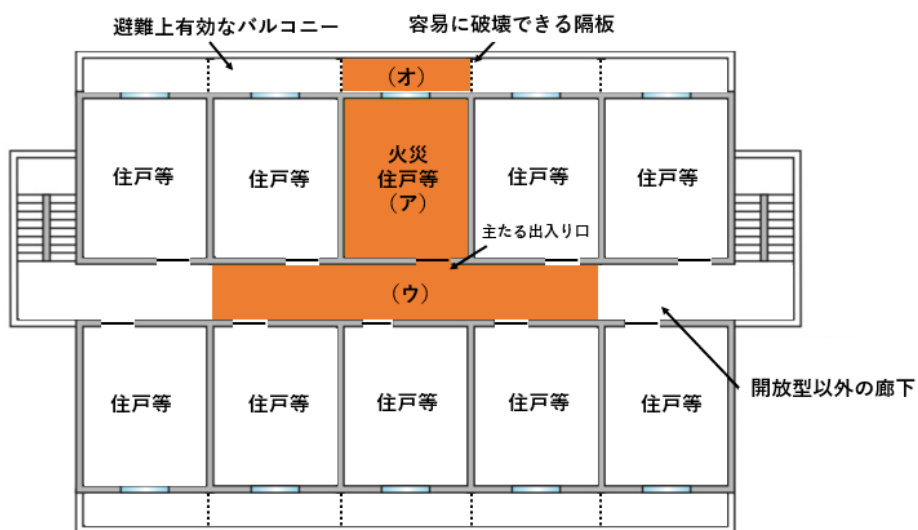
第4-5図 (廊下型特定共同住宅等 (中廊下型で連続したバルコニー))
