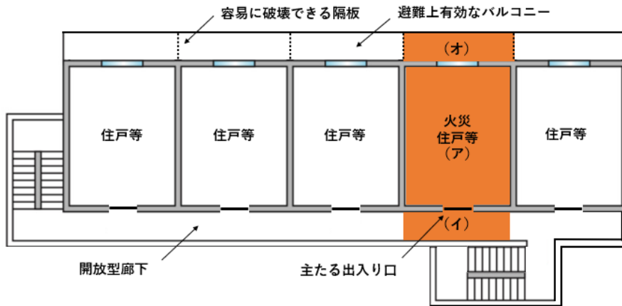
第4-3図 (廊下型特定共同住宅等 (連続したバルコニー、2の階段のうち1が端部に存する場合))
