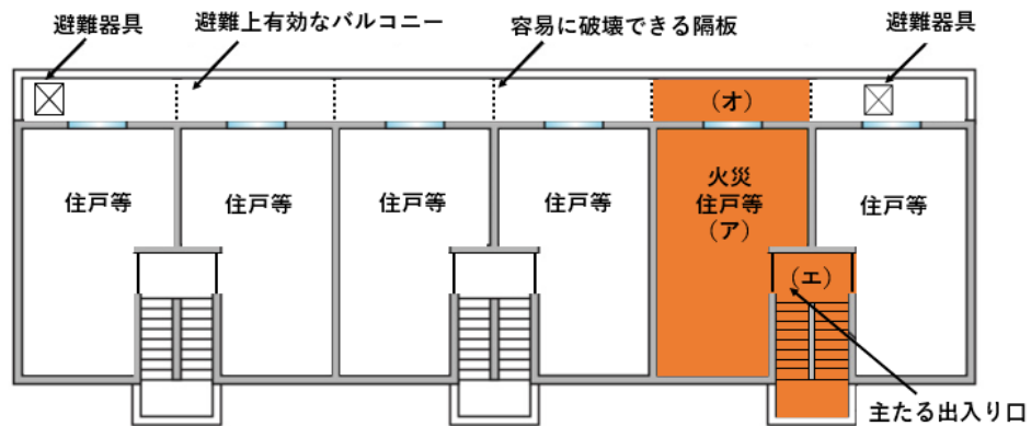
第4-6図 (階段室型特定共同住宅等 (連続したバルコニー))
