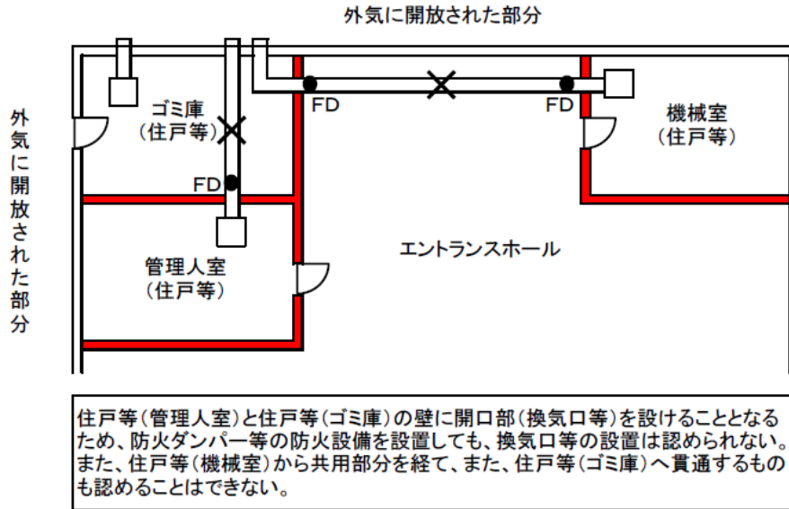
第3-20図 (認められない設置例)
