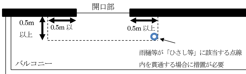
第3-22図 (ひさし等を貫通する配管の防火措置)
