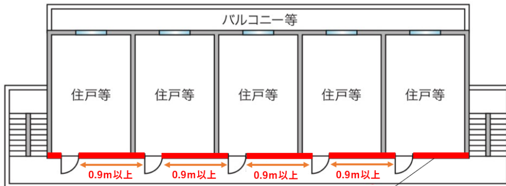
住戸等と共用部分を区画する壁を示す 【位置・構造告示第3第3号(3)】
