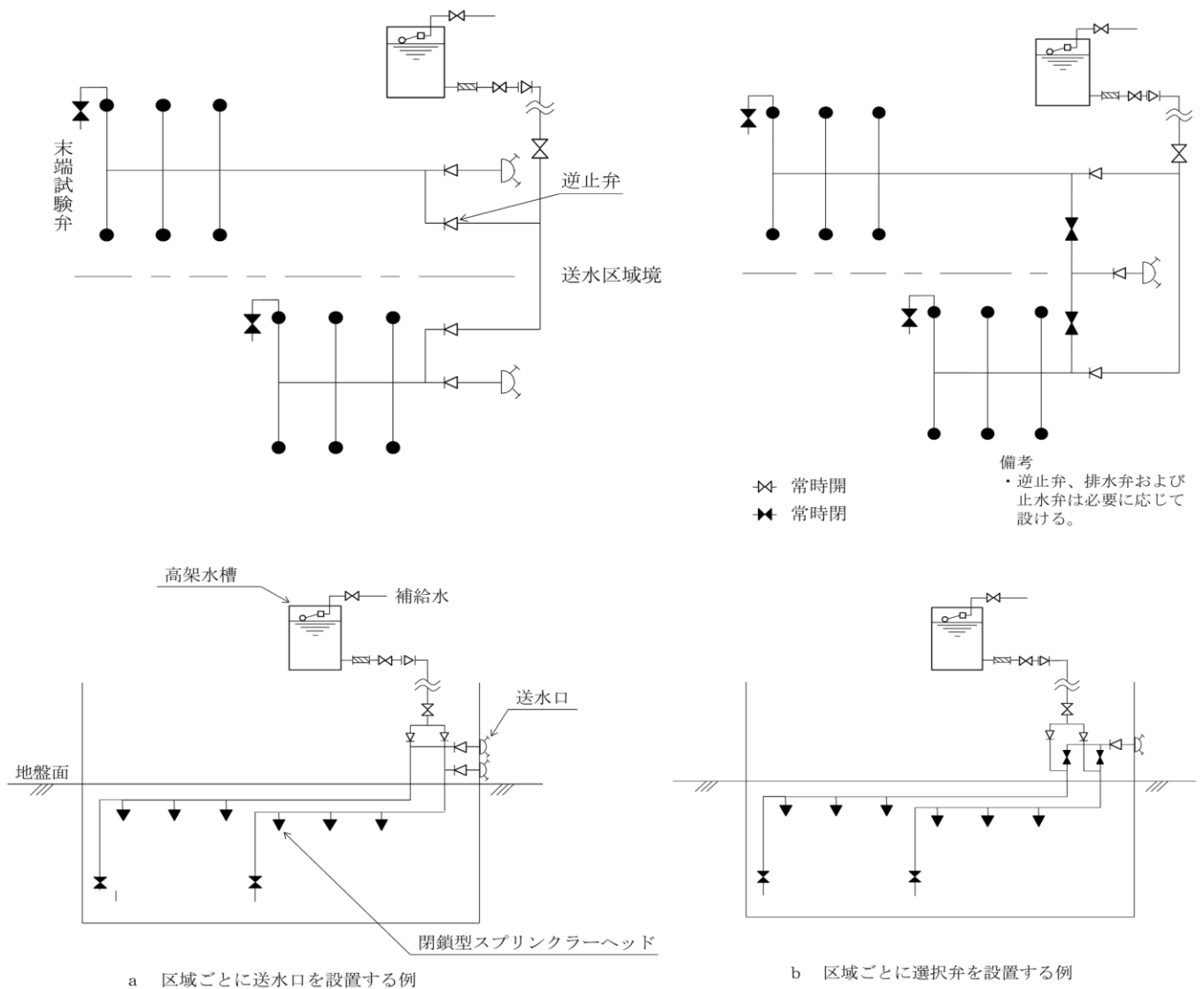
第21-2図 閉鎖型スプリンクラーヘッドを用いる方式の構成・系統図例 (配管内を常時充水する場合)
