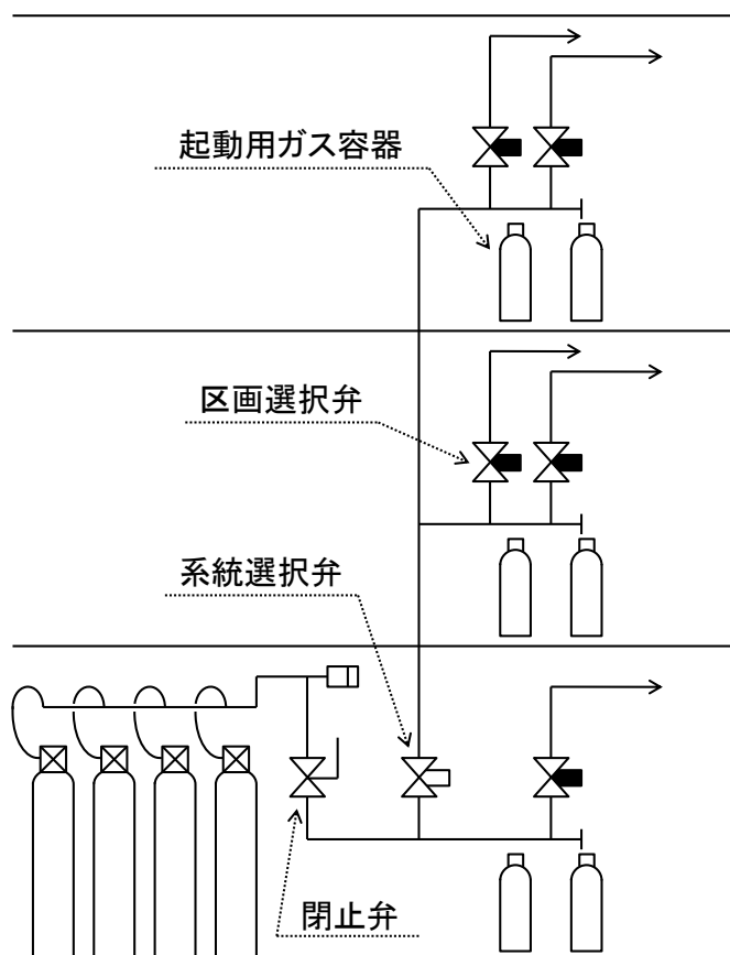
第7-5図 複数の選択弁（系統選択弁・区画選択弁）を経由する例
