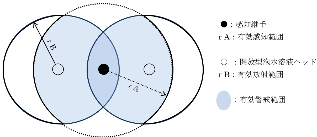
第26-4図（平面図）
