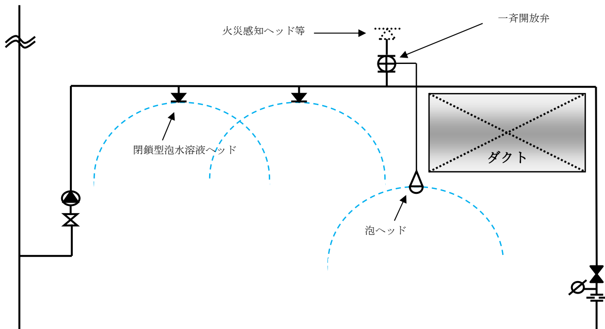
第26—7図（構成例）
