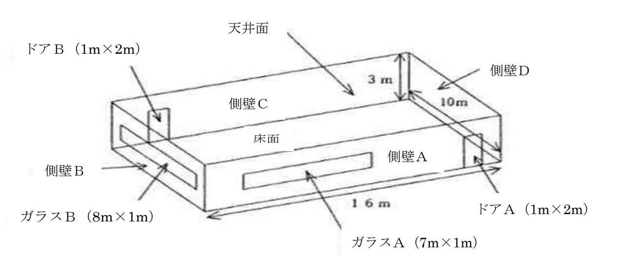
【図1】室概要
