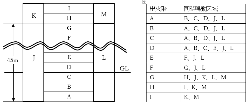
第16-15図 区分鳴動方式の概念図
