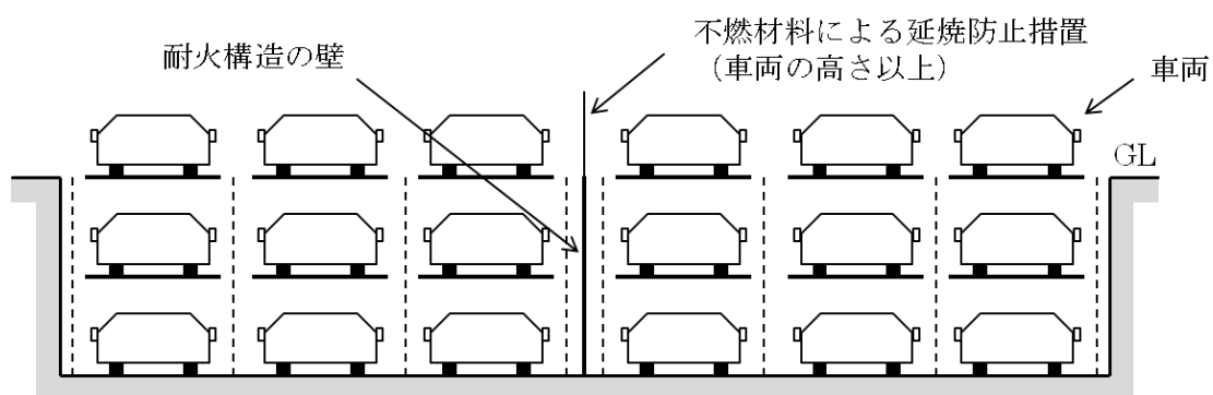
(断面図)
