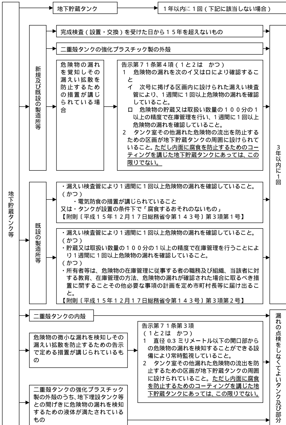
別図 1 3 [地下貯蔵タンク・FRP外殻]
