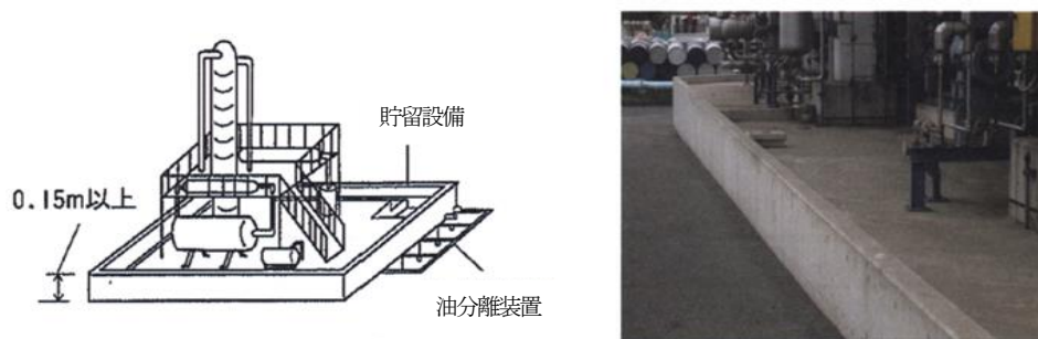
屋外設備の囲い等の例
