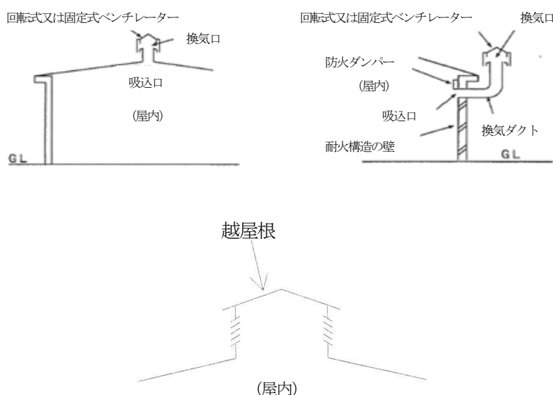
換気・排出設備の例
