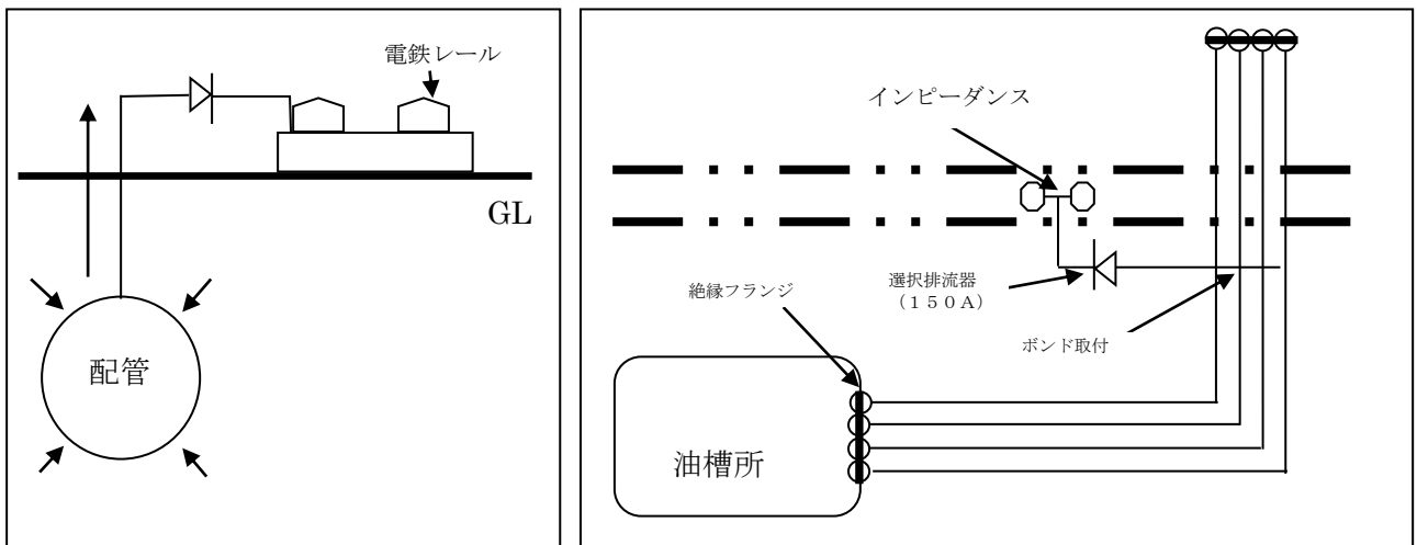
図6 排流法
