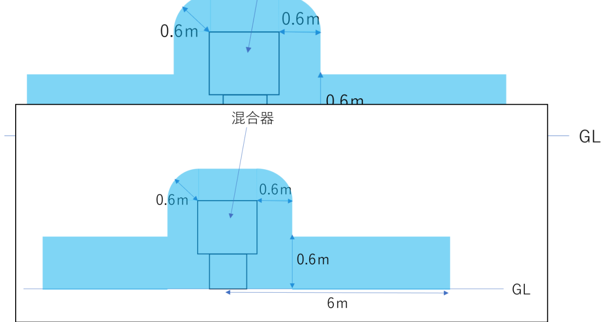
図5 混合燃料調号器の周囲の可燃性蒸気滞留範囲※
