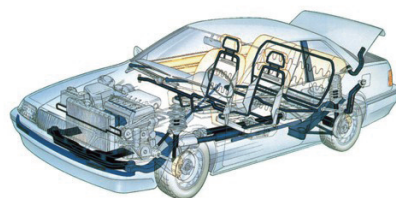
自動車部品としての鋼管使用例
