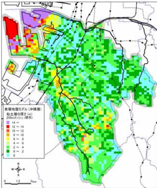
(a) 粘土層
