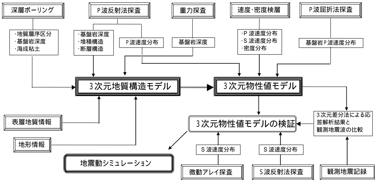
図 2.3-2 3次元地盤モデルの作成手順（大阪府，2005）
