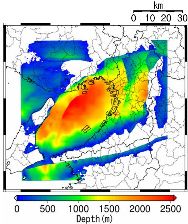
図 2.3-1 基盤岩深度構造モデル（大阪府，2005）
