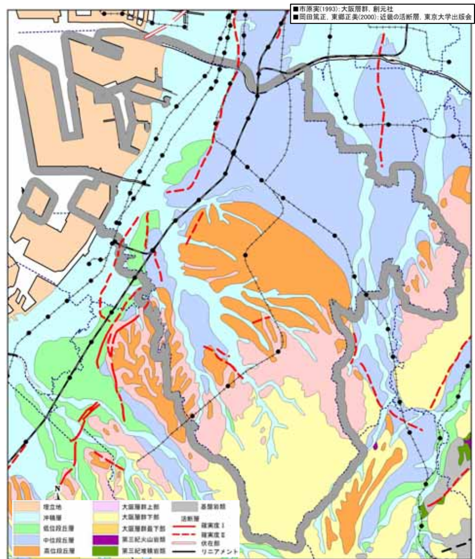
図 2.1-3 表層地質図
