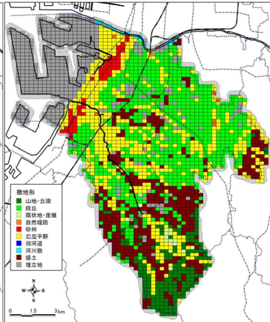
図 4.2-5 微地形区分 (250m メッシュ)
