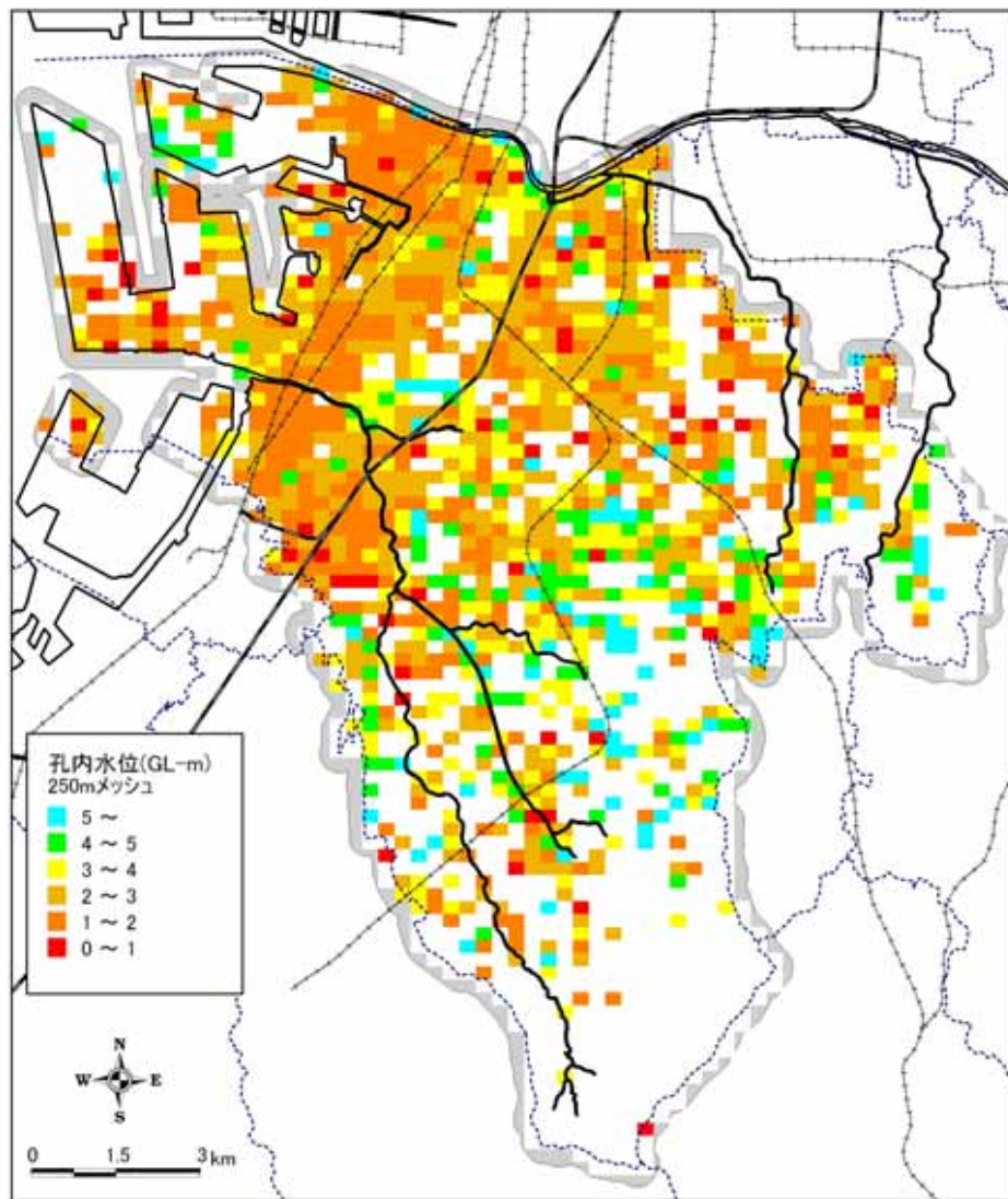
図 4.2-4 平均孔内水位 (250m メッシュ)
