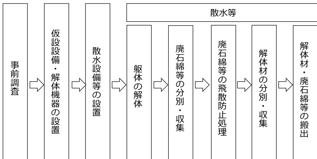
図7.1 注意解体の標準手順におけるアスベスト飛散防止措置の実施工程
