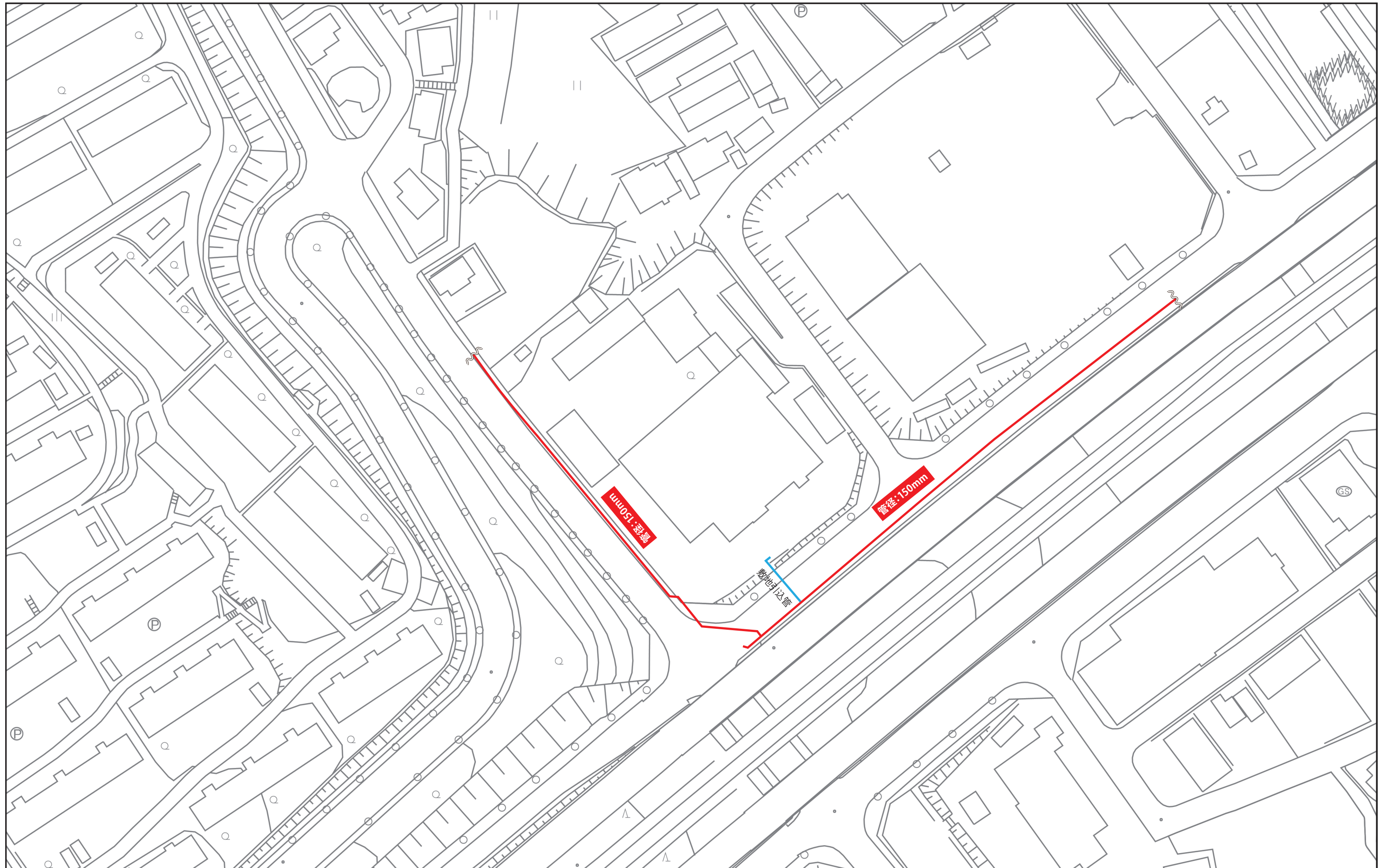
敷地周辺インフラ現況図 上水管
