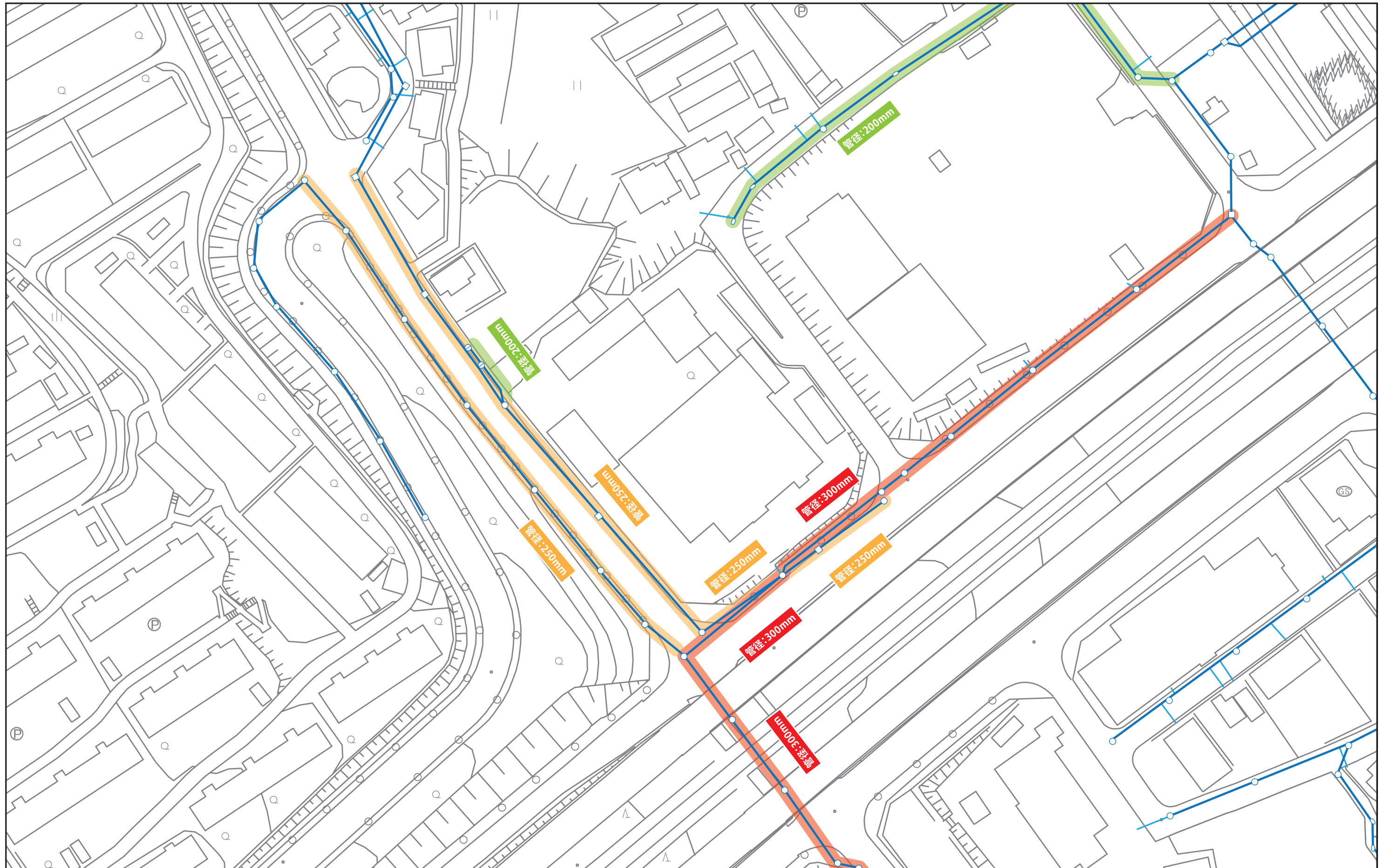
敷地周辺インフラ現況図 下水管-汚水
