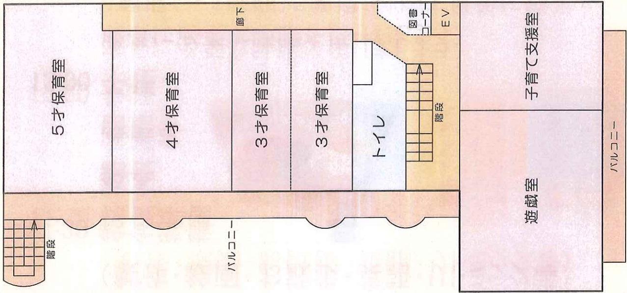
2階平面図
