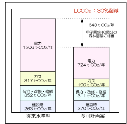
従来水準型と今回計画のライフサイクルCO2の比較
