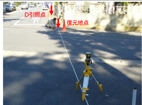
C引照点での基準器による視準(C引照点～復元地点～D引照点)
