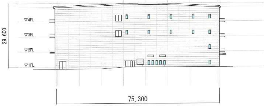
南立面图
