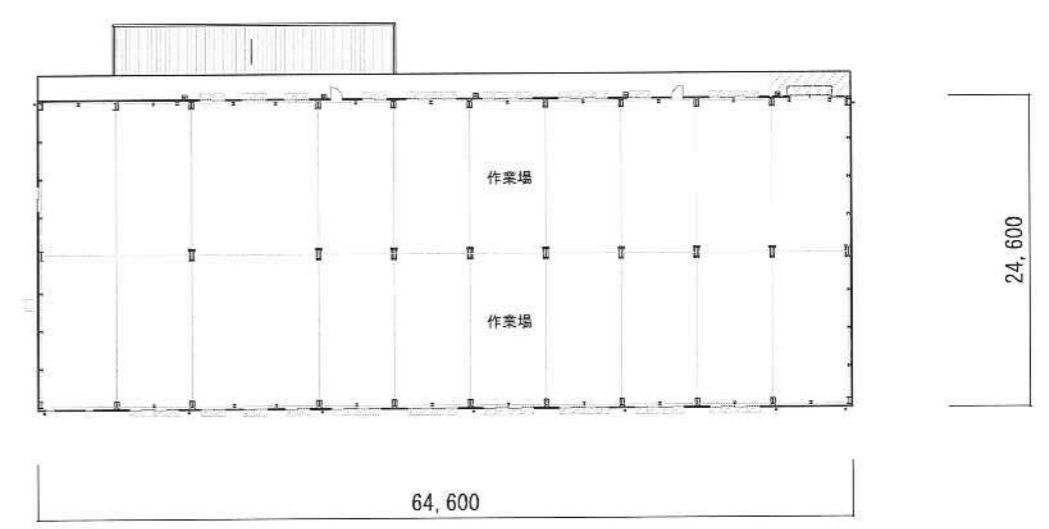
2階平面図
