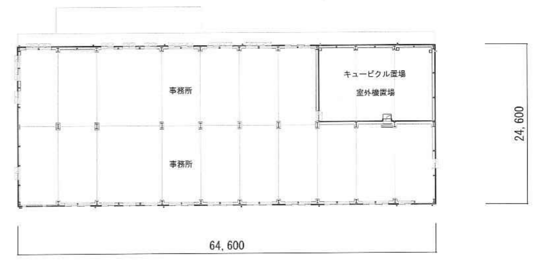
3階平面図
