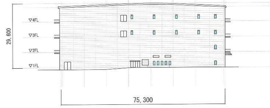
南立面图
