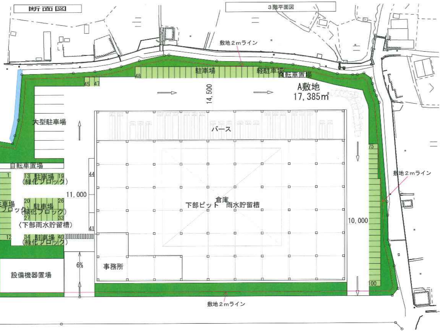
1階平面図
