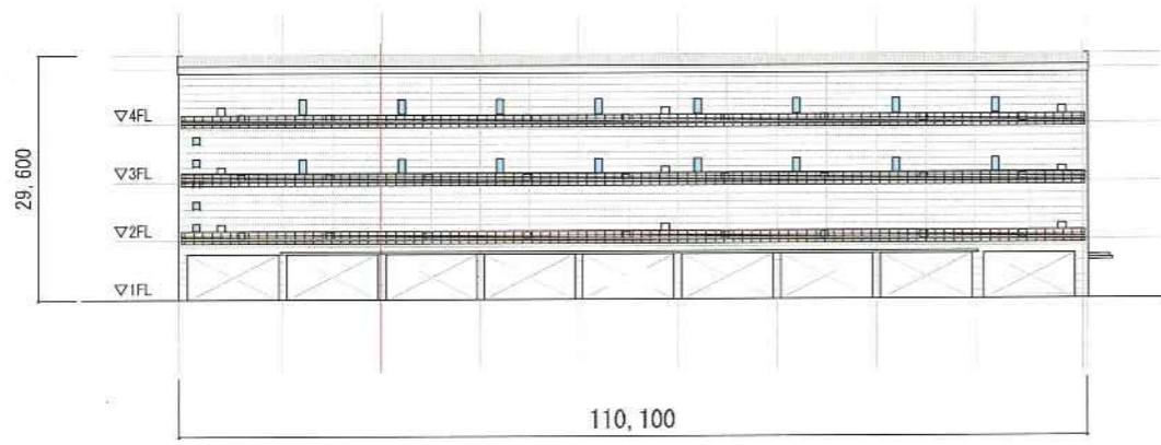
東立面图
