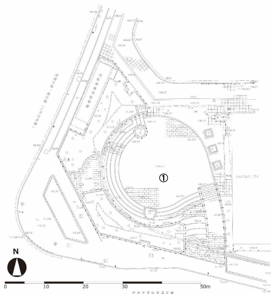
■新金岡町ブリック公園現況施設図
