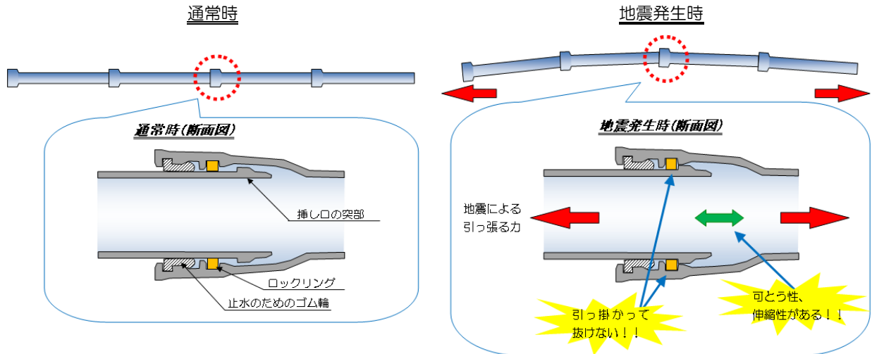
図表 4-6-2 耐震管のイメージ
