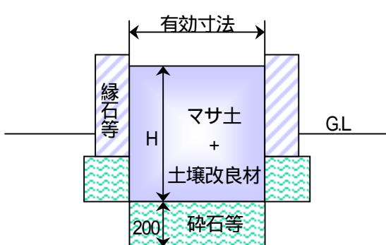
土壌断面図(標準断面)
