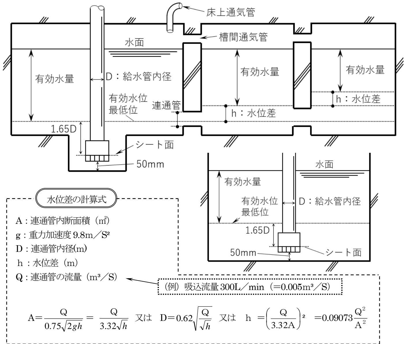
第2-8図 サクションピットを設けない場合又は連通管を設ける場合
